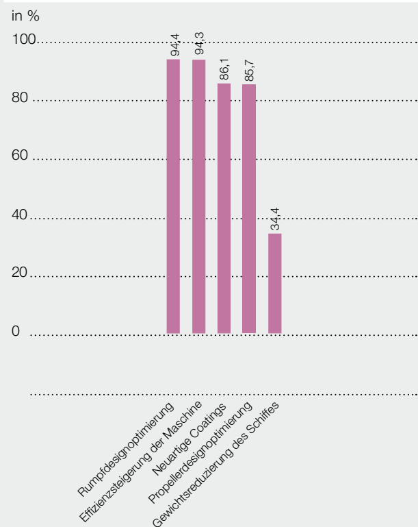
Mit welchen technischen Möglichkeiten kann die Milage (Reichweite pro Tonne Bunkerverbrauch) der Schiffe erhöht werden? (Abb. 6)
