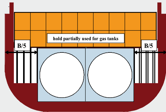
Querschnitt eines gasbetriebenen Containerfeederschiffs (Abb. 3)
